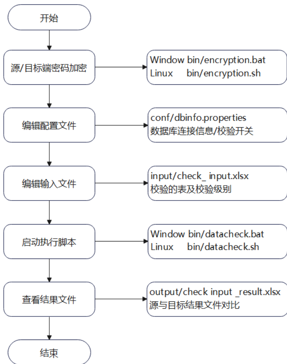
图 7-1 DataCheck 流程图
